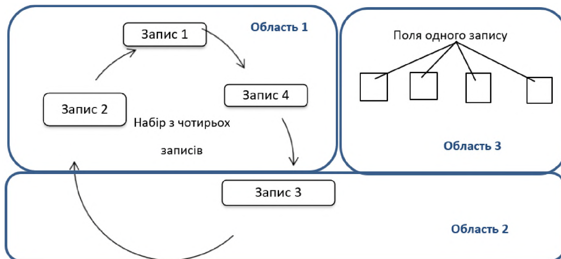
Рис. 5. Структура мережної бази даних.
