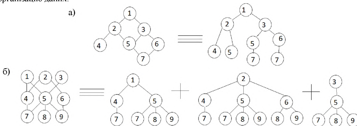
а) у вигляді одного дерева; б) у вигляді об'єднання дерев.
